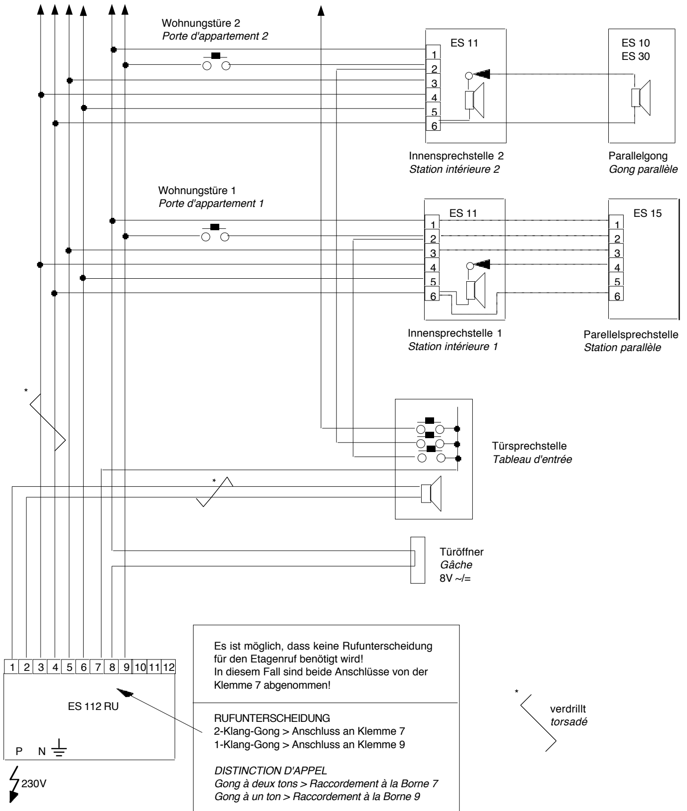
Türsprechanlage ESAG Typ 100 (ES112 RU)
